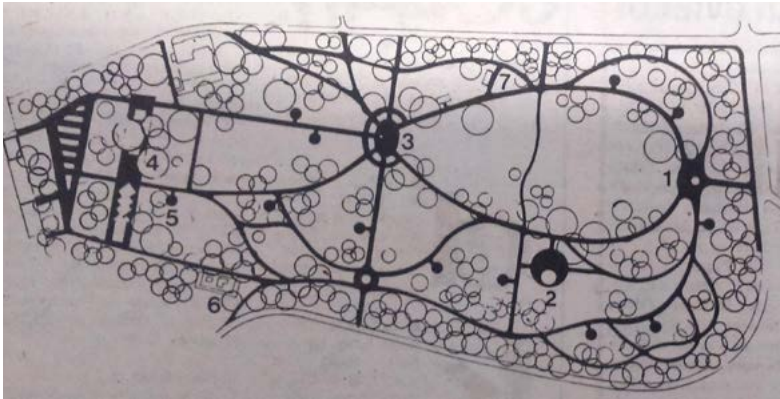
68 • Pôdorys Sadu Janka Kráľa po rekonštrukcii. Pohľad z juhu (od diaľnice). 1. Gotická veža; 2. Odpočinková plocha s fontánou; 3. Centrum parku so sochou Janka Kráľa; 4. Objekt pre správu s občerstvením a terasou; 5. Jedno z odpočívadiel; 6. Detské ihrisko; 7. Čerpacia stanica a sociálne zariadenie.
